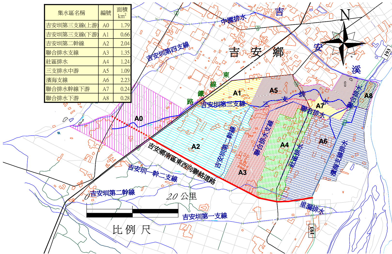
圖 2-2 聯合排水系統子集水區面積圖
